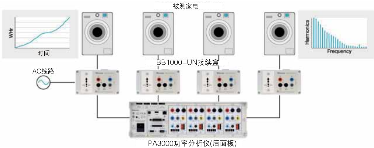
家测试电和消费电子的测试配置和测量结果实例
